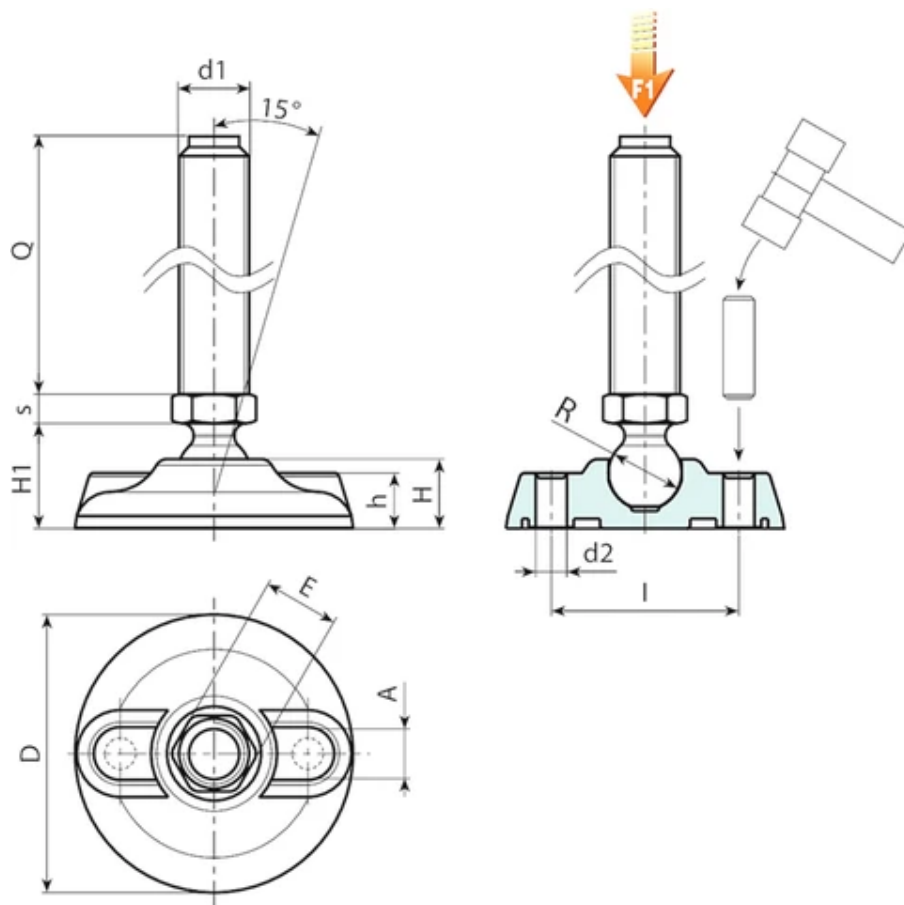
Версия P902: Опора со стержнем типа А (с шестигранником) и шаровой головкой 15
