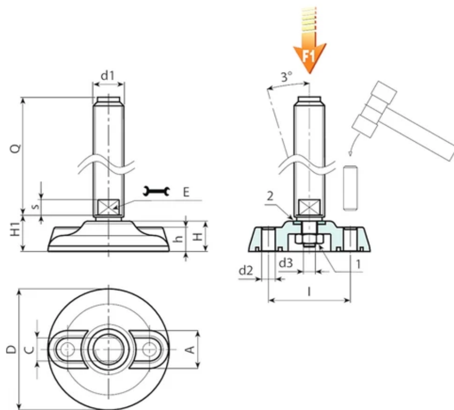
Версия P800: Опора с вращающимся стержнем, крепление с помощью гайки.
