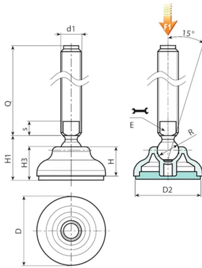
Versão P910: Pé de apoio com perno tipo B (alojamento para chave fresado) e esfera 15 - com antiderrapante em SBS
