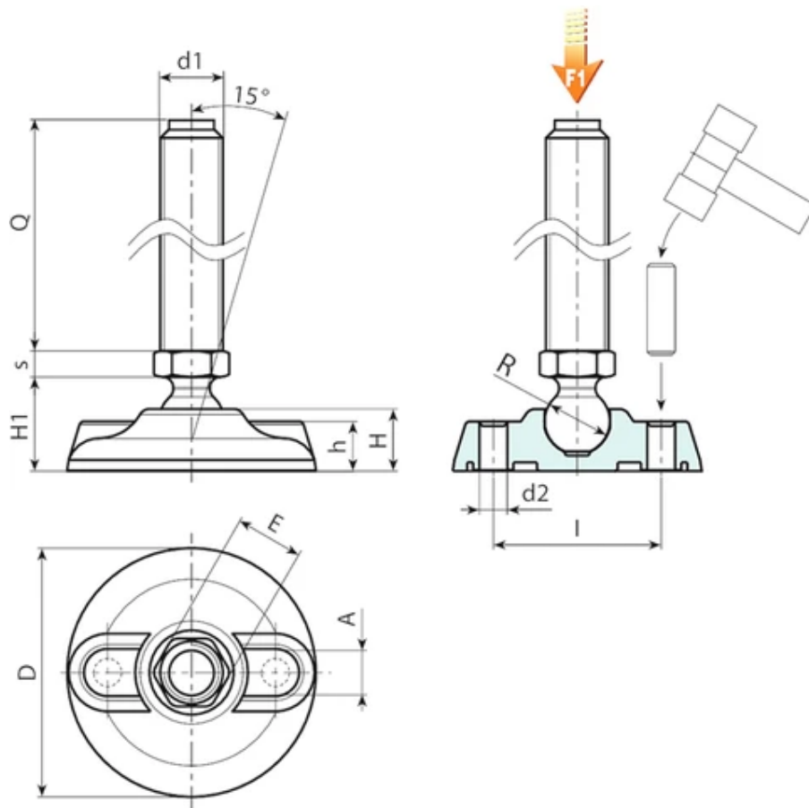
Versão P902: Pé de apoio com perno tipo A (com hexágono) e esfera 15
