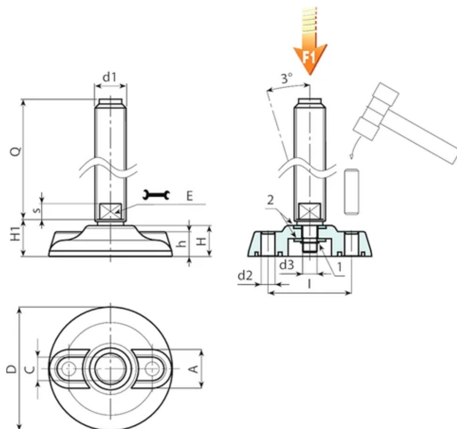
Versão P801: Pé de apoio com perno rotativo com fixação por meio de Seeger
