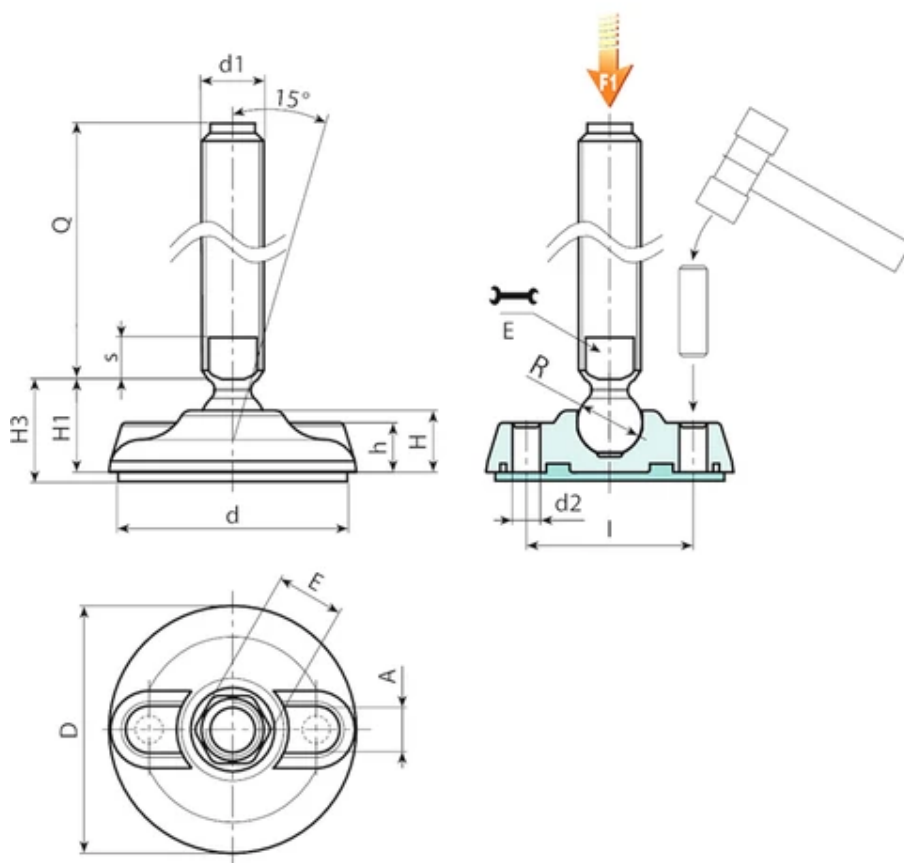
Wersja P917: Stopka podporowa z trzpieniem typu B (z frezowanym gniazdem pod klucz) i kulka 15 - z podstawą antypoślizgową z SBS
