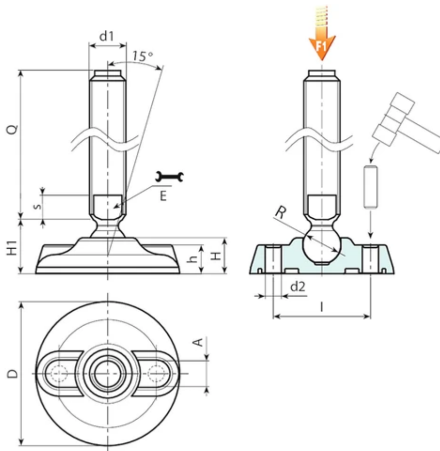
Wersja P914: Stopka podporowa z trzpieniem typu B (z frezowanym gniazdem pod klucz) i kulką 24
