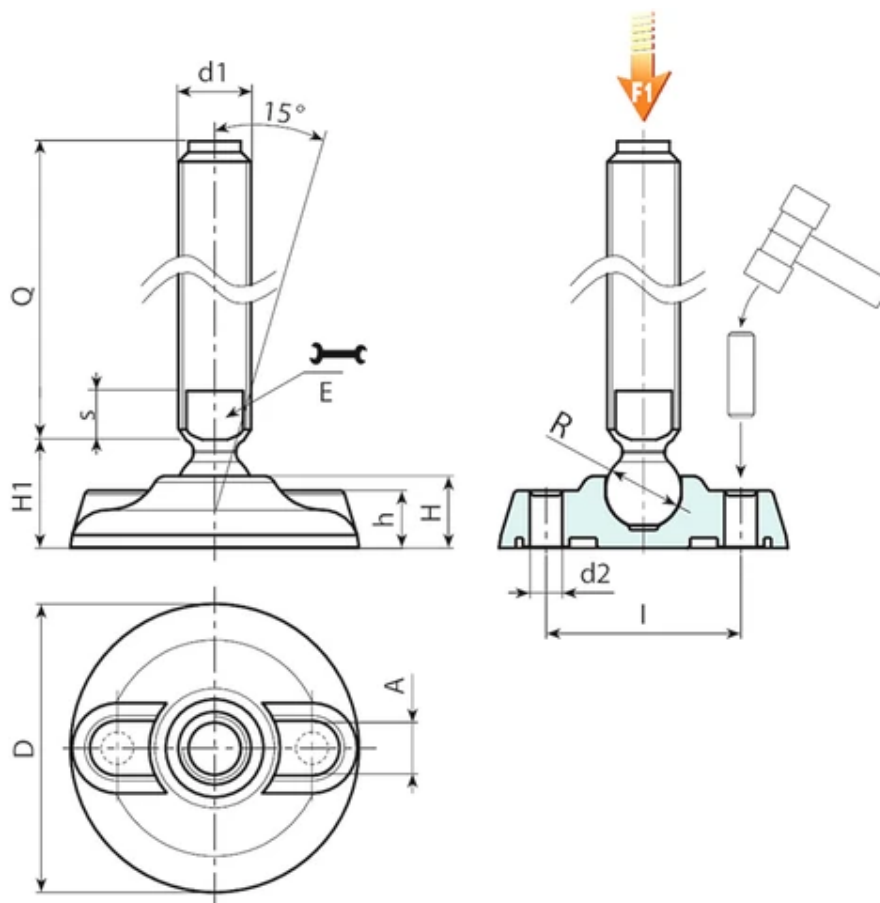
Wersja P913: Stopka podporowa z trzpieniem typu B (z frezowanym gniazdem pod klucz) i kulką 15
