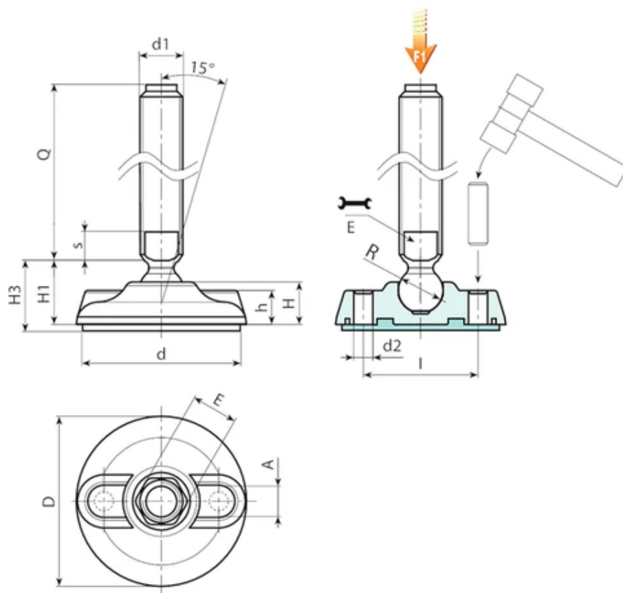
Versie P917: Stelvoet met draadeind type B (gefreesde zitting voor moersleutel) en kogel 15 - antislipschijf in SBS.
