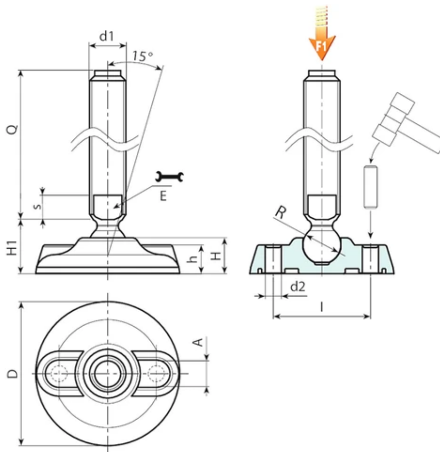
Versie P914: Stelvoet met draadeind type B (gefreesde zitting voor moersleutel) en kogel 24
