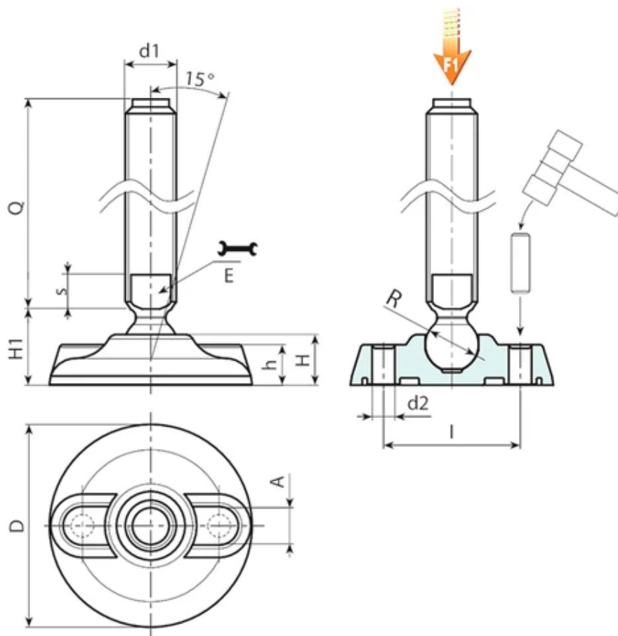
Versie P913: Stelvoet met draadeind type B (gefreesde zitting voor moersleutel) en kogel 15.
