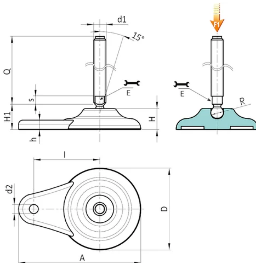
Versie P708: Stelvoet met laterale bevestiging met draadeind type B (gefreesde zitting voor moersleutel) en kogel 24.
