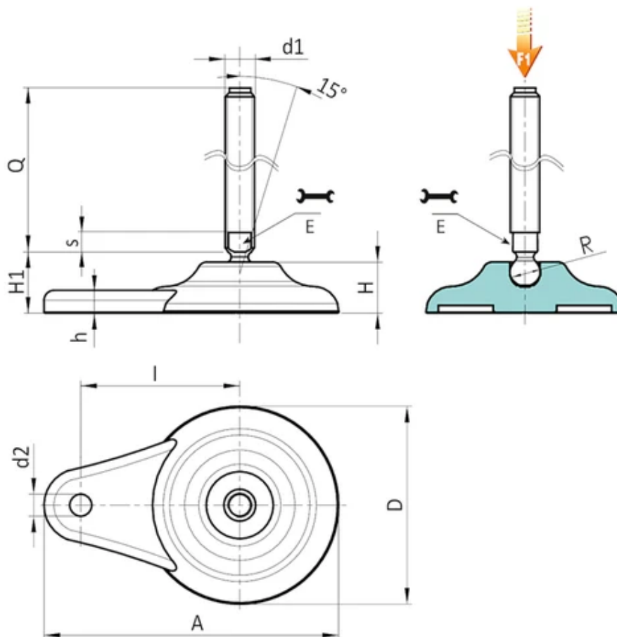
Versie P706: Stelvoet met laterale bevestiging met draadeind type B (gefreesde zitting voor moersleutel) en kogel 15.
