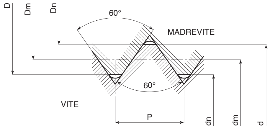
Madrevite UNC con tolleranza 2B
