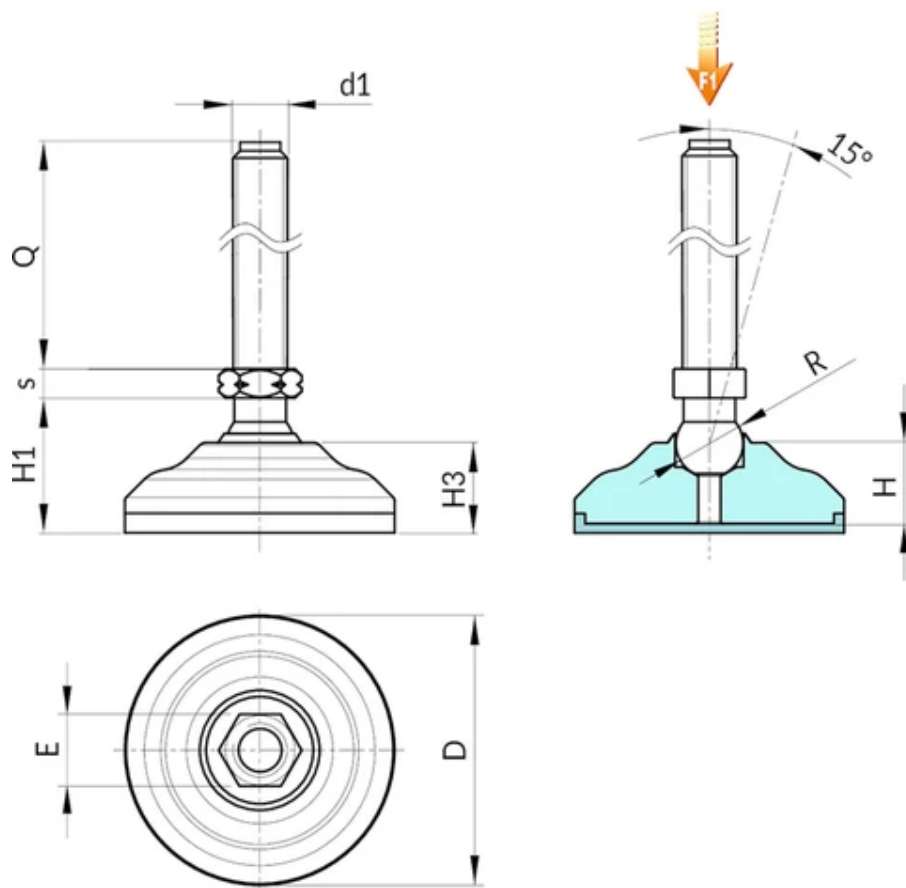
P544 változat: Horgonyzott acél rögzítőláb A típusú szárral (hatszögletű talppal) és 24 golyóval - TPV csúszásmentes talppal
