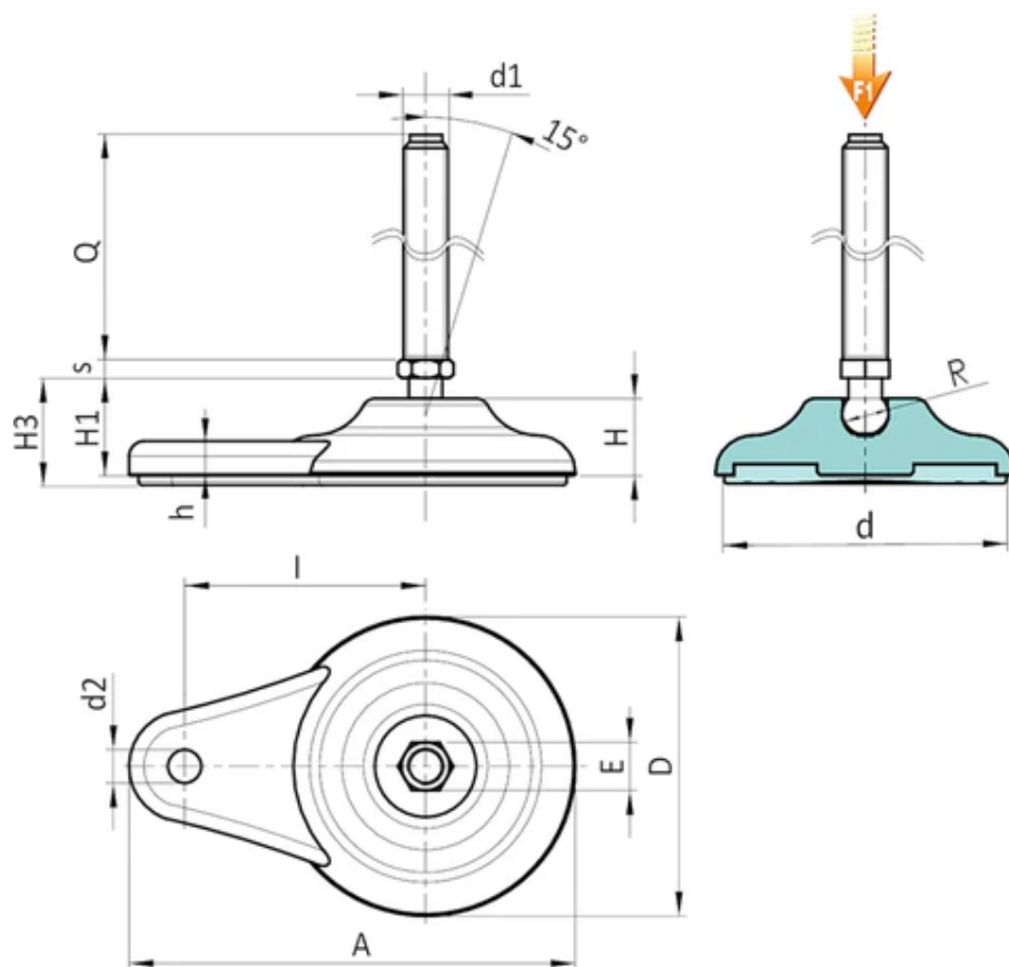
Versio P703: Tukijalka, sivukiinnitys, A-tyyppinen varsi (kuusiomainen alusta) ja pallo 15 - luistamisenesto SBS-kumia
