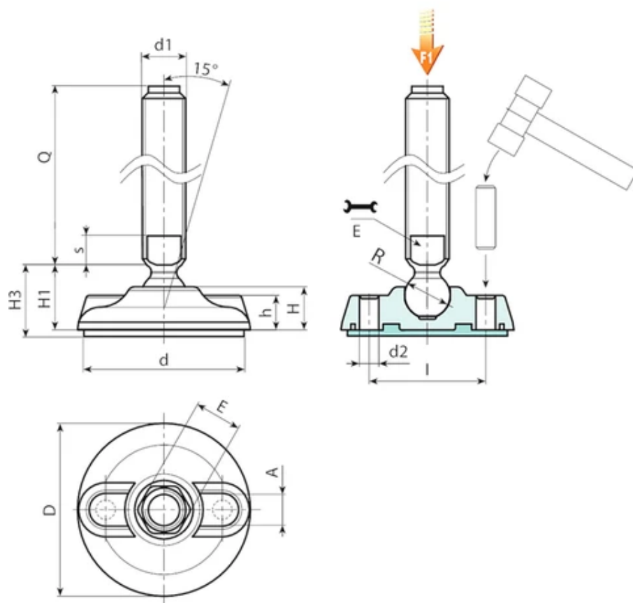
Versión P918: Pie de apoyo con perno tipo B (alojamiento fresado para llave) y bola 24 - con base antideslizante de SBS
