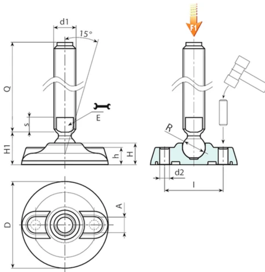
Versión P913: Pie de apoyo con perno tipo B (alojamiento fresado para llave) y bola 15
