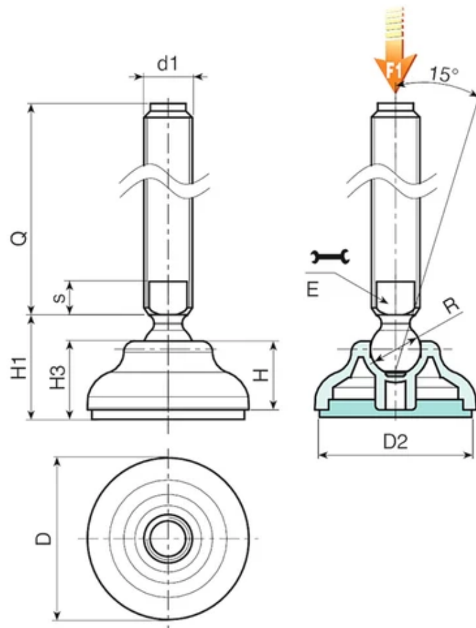
Ausführung P909: Gelenkfuß mit Verstellspindel Typ B (mit Aufnahme für Gabelschlüssel) und Kugel 12,4 - mit rutschfester Gummiauflage aus SBS
