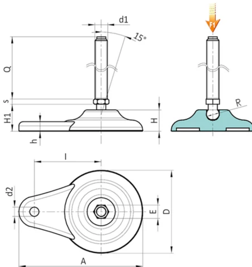
Version P702: Støttefod med sidefastspænding, skafttype A (med sekskant) og kugle 15
