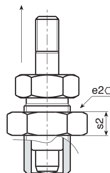
Êmbolo em posição recuada
