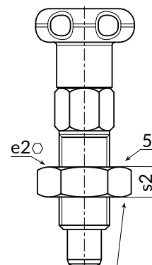
Tuerca de bloqueo solo con versión W736CIN
