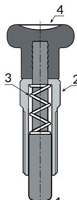
Émbolo de indexación en posición retraída
