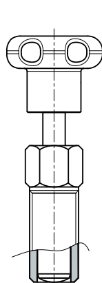
Émbolo de indexación en posición retraída
