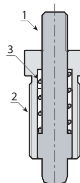
Dugattyú visszahúzott pozícióban
